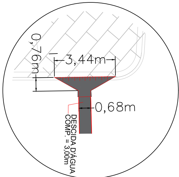
DETALHE - ENTRADA P/ DESCIDA D'ÁGUA (EDA 02 B) - 1/25
