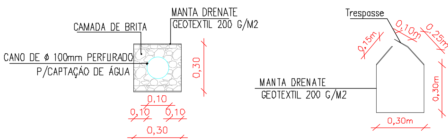
DETALHE – 01 DETALHE DA VALA DO TUBO DE DRENAGEM
