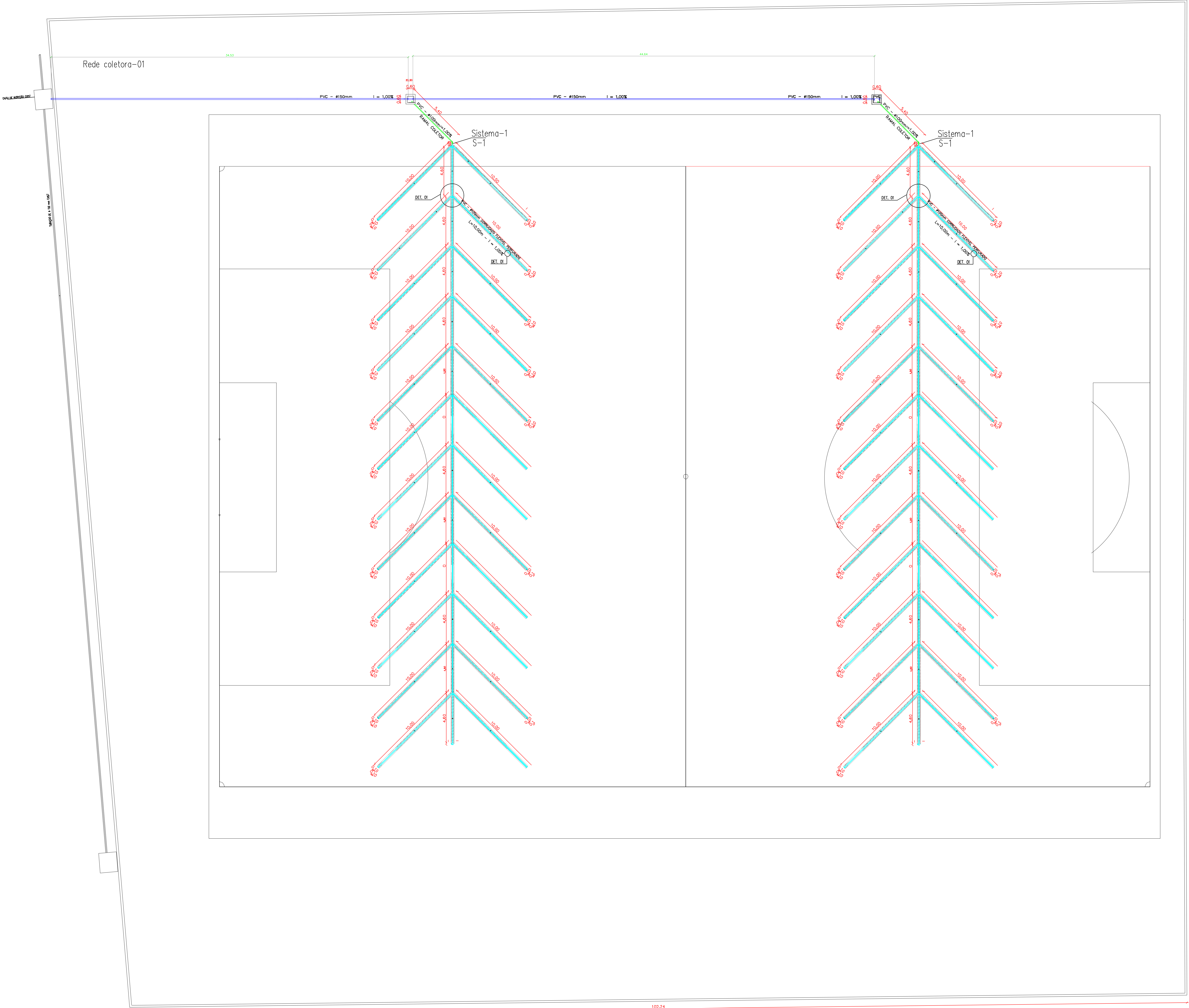
PLANTA BAIXA ESC 1/150
